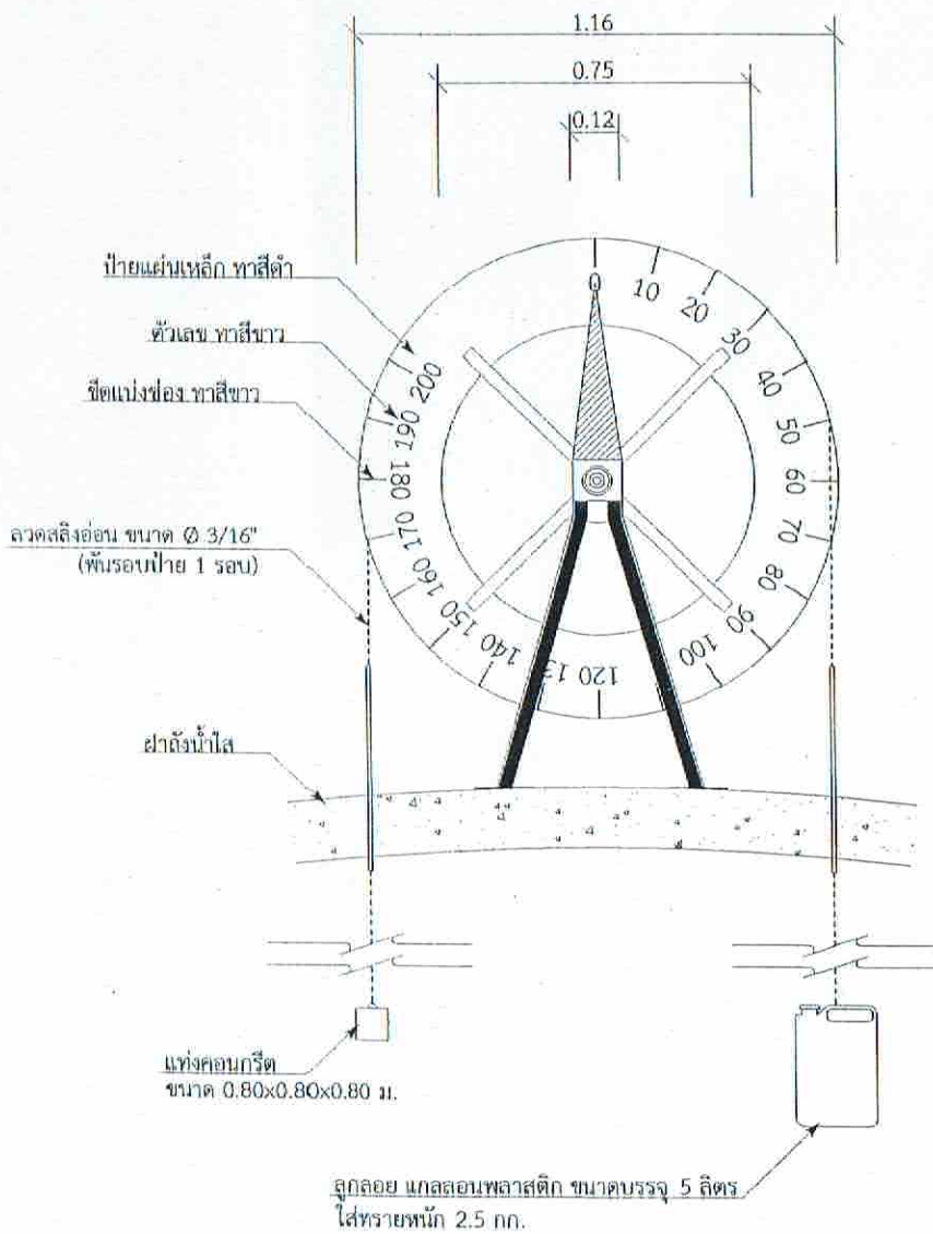
รูปด้านหน้า ป้ายบอกระดับน้ำ(ถังน้ำใส)
