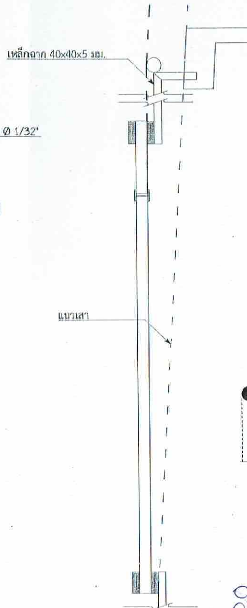
แบบป้ายบอกระดับน้ำ(หอดังสูง)
