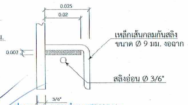
รูปขยาย 4
