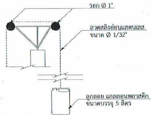
แบบขยาย รอก(หอดังสูง)
